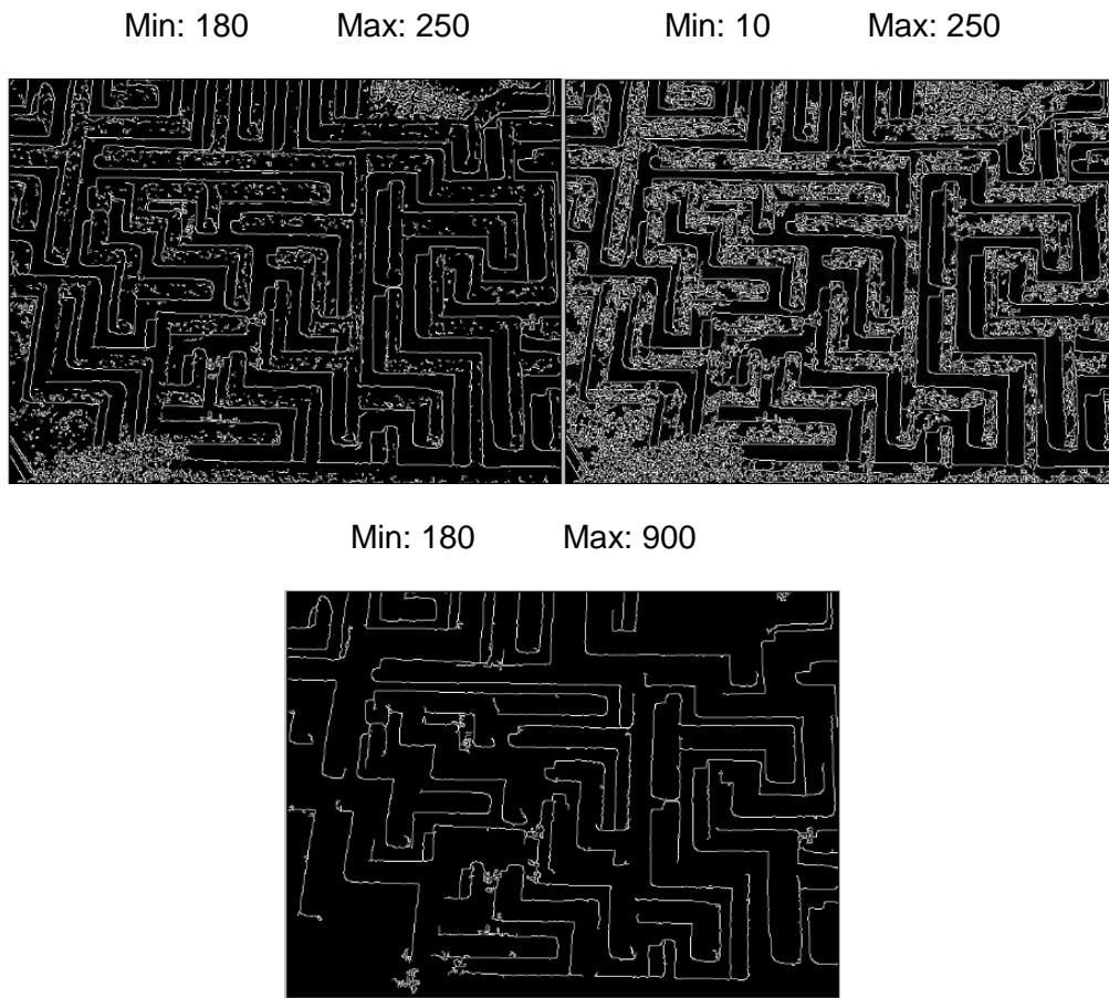
Figure 22 Edge Detection
